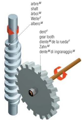
engrenage M à vis F sans fin F worm gear engranaje M de tornillo M sin fin M Schneckengetriebe N ruota F elicoidale
